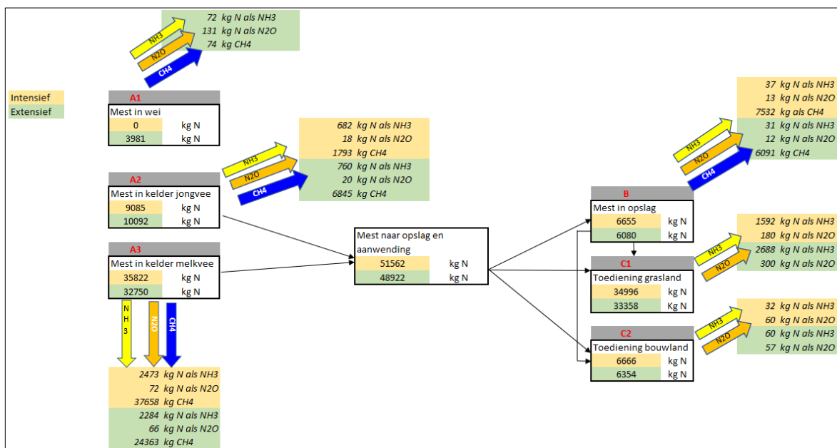
Figuur B3.1 Scenario 1: Regulier geen vergisting.
