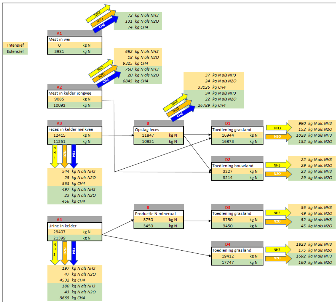
Figuur B3.10 Scenario 9.1: Semi-dichte vloer + onder afzuiging + strippen.
