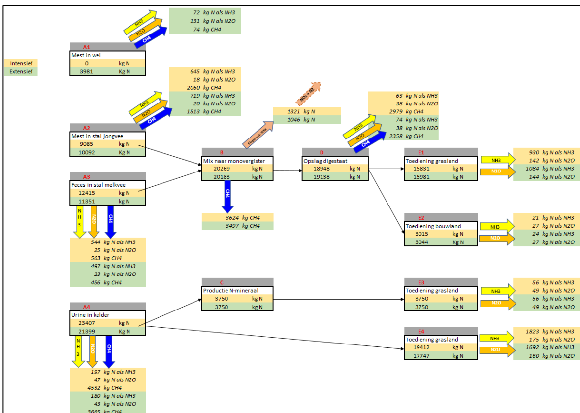
Figuur B3.11 Scenario 9.2: Semi-dichte vloer + onder afzuiging + strippen + monovergisten.
