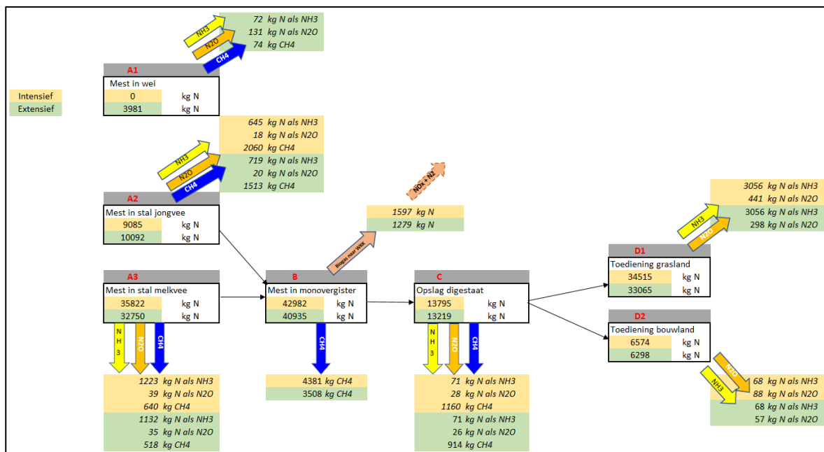
Figuur 3.2 Voorbeeld schematische weergave voor berekening emissies (In bijlage 3 zijn de schematische weergaven van alle scenario's weergegeven).
