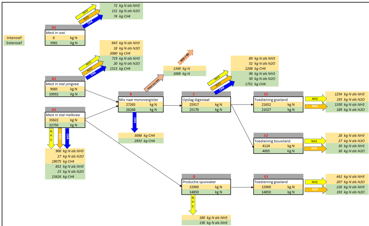
Figuur B3.5 Scenario 4.2: Regulier + verdunnen + monovergisten + strippen.
